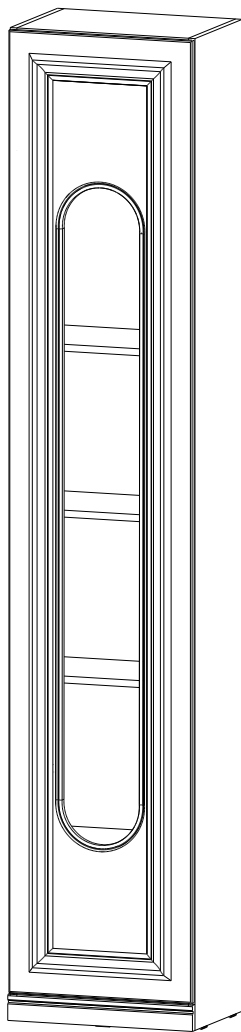
Пенал открытый (450*332*2288)
